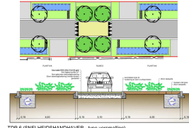
TOP 6 (SNELHEIDSHANDHAVER - type versmalling)
