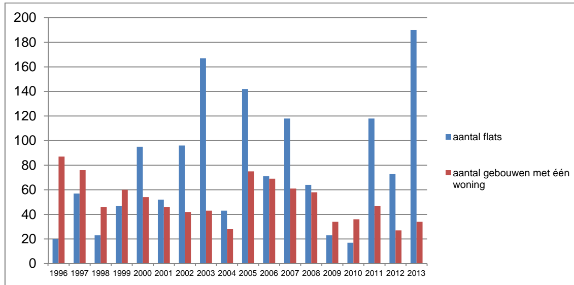
Figuur 21: grafiek met vergelijking aantal verleende bouwvergunning voor aantallen flats versus aantallen gebouwen met één woning (gebaseerd op data van algemene directie van statistieken)
